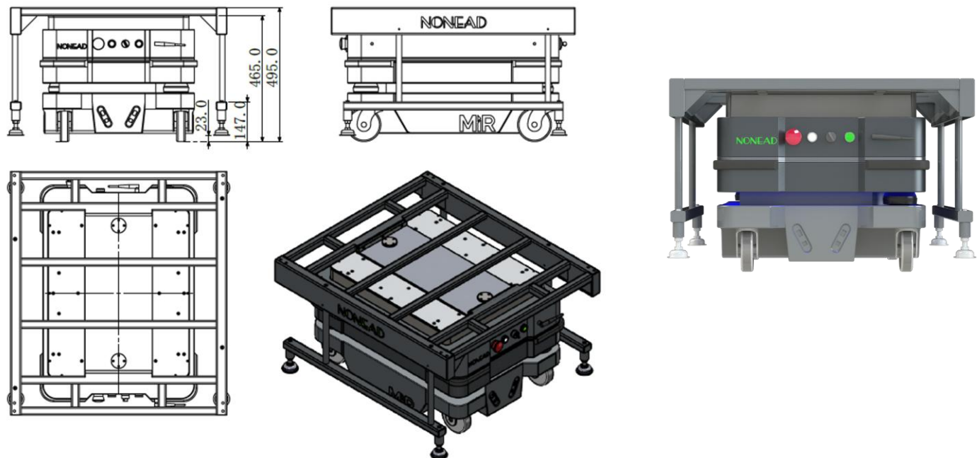
基准料架举升尺寸图
