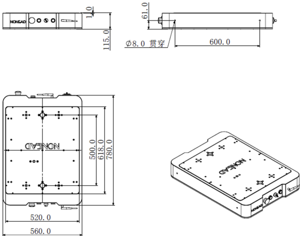
NH0398 第四代拓德顶部举升系统 待机尺寸 单位: mm
