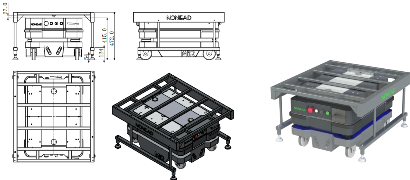
基准料架举升尺寸图
