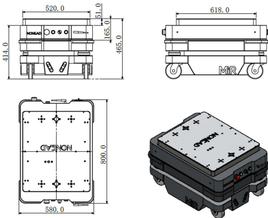
安装了 NH0398 第四代拓德顶部举升系统的 MiR250 举升状态
