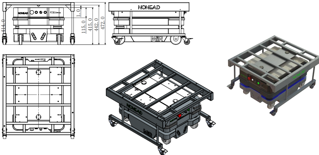
基准料车举升尺寸图
