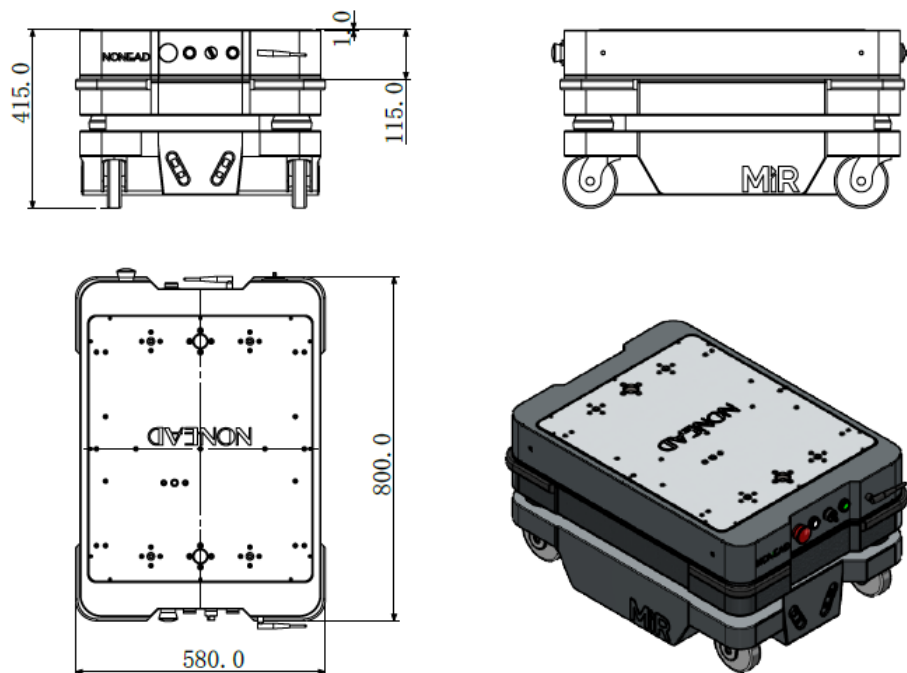
安装了 NH0398 第四代拓德顶部举升系统的 MiR250 待机状态
