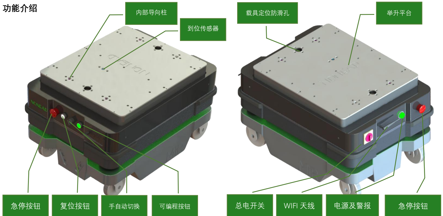
第四代拓德顶部举升系统功能按钮介绍
