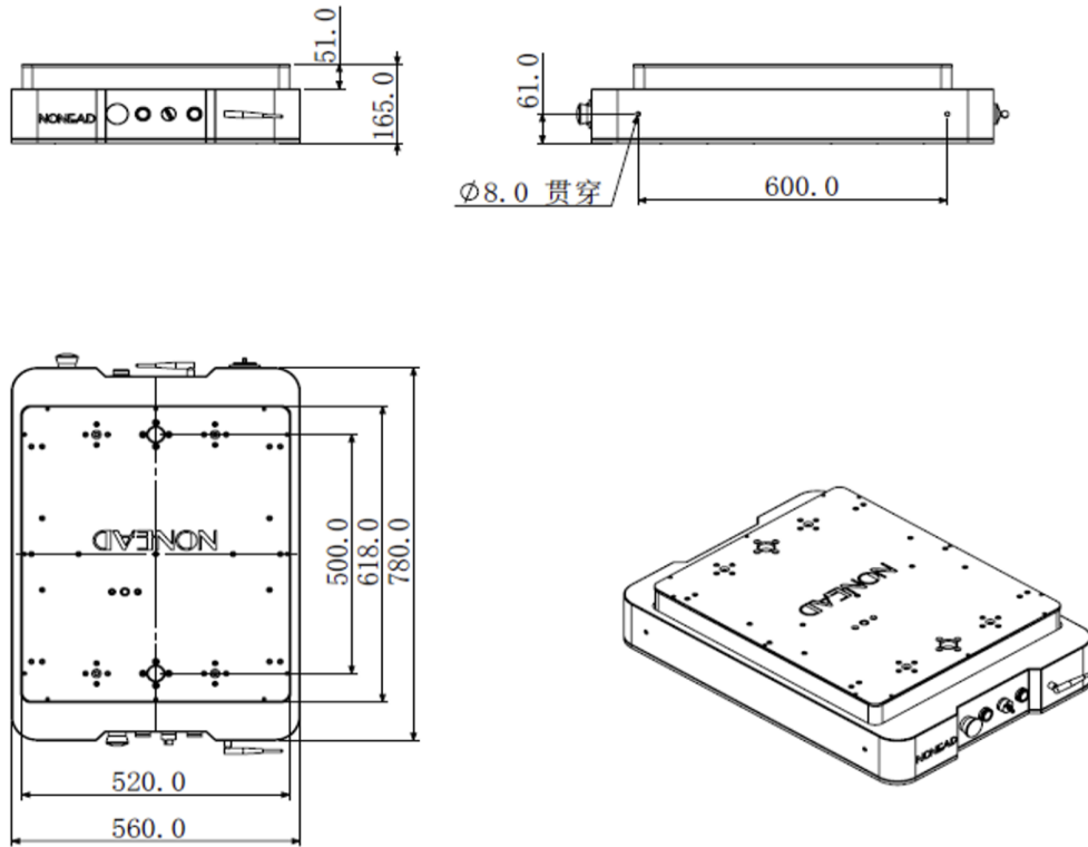
NH0398 第四代拓德顶部举升系统 举升尺寸 单位: mm
