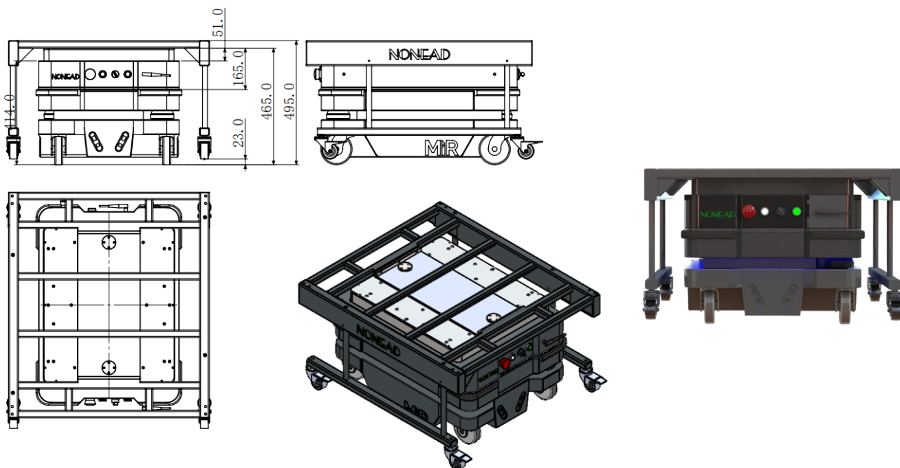
基准料车举升尺寸图
